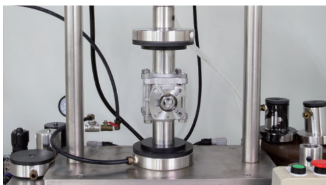
ISO 15848-1 測試
